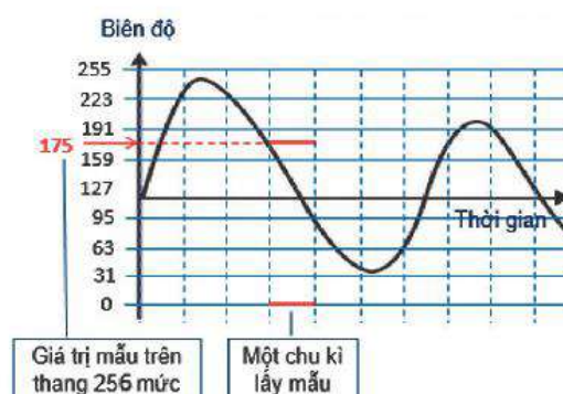
Hình 6.2. Chu kì lấy mẫu và thang giá trị mẫu
